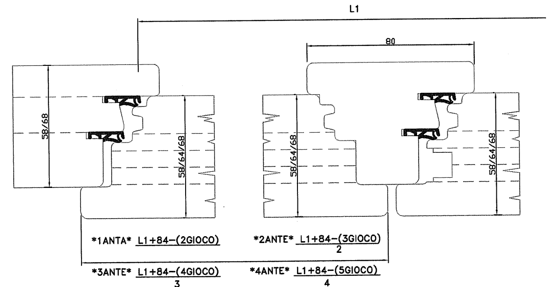
SEZIONE ORIZZONTALE CON PILASTRINO
