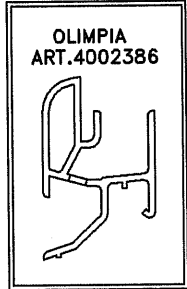
SEZIONE VERTICALE
