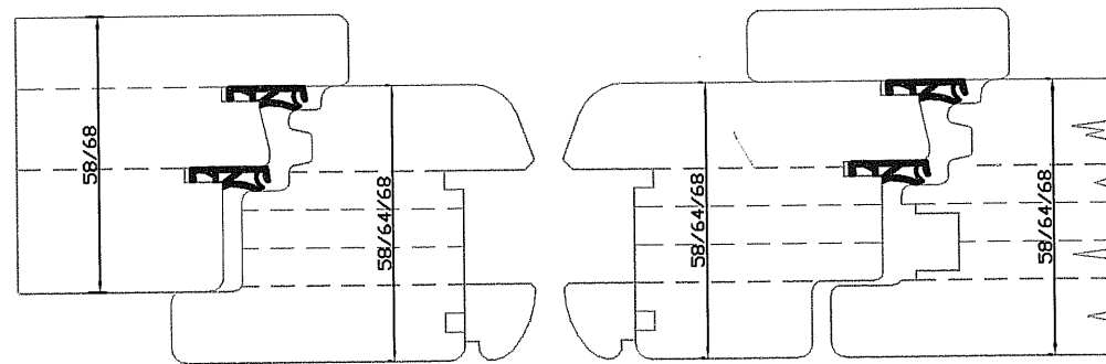
SEZIONE ORIZZONTALE
